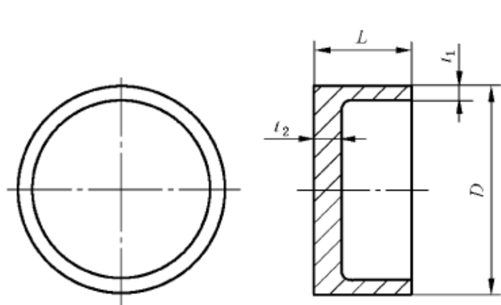
图 4 碗形锻件 ( L \leq D )
