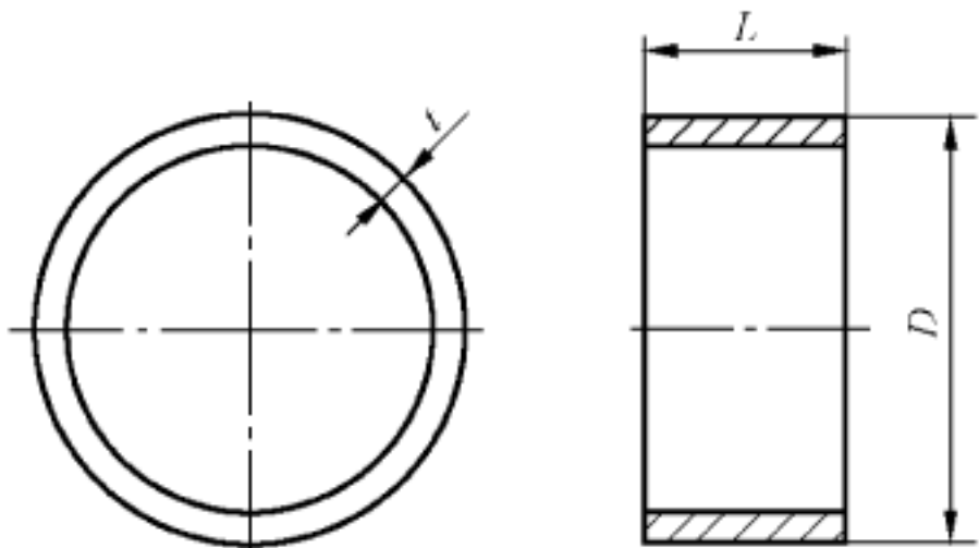
图 2 环形锻件 ( L \leq D )
