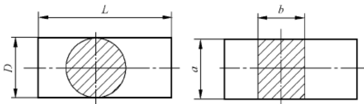
图 6 条形锻件
